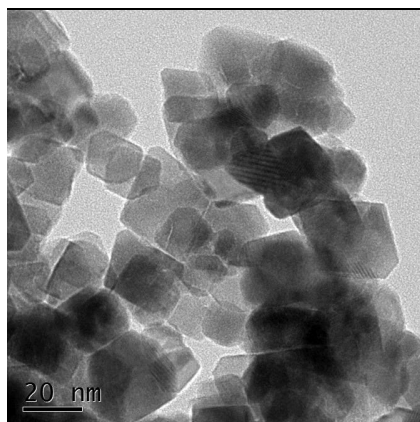
纳米氧化铈电镜图
