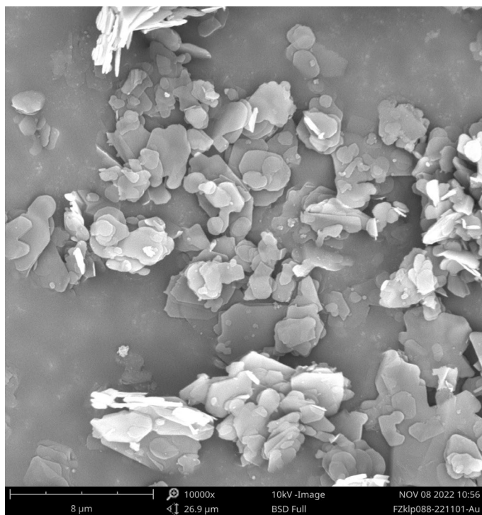
( N-3 电镜图)
